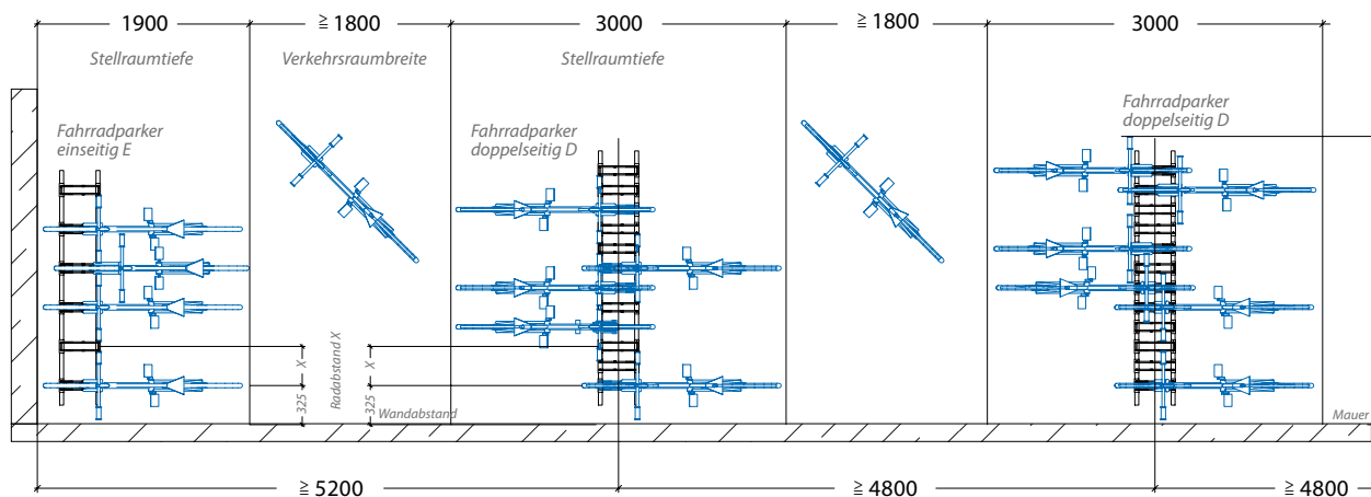
PLANUNGSSKIZZE
